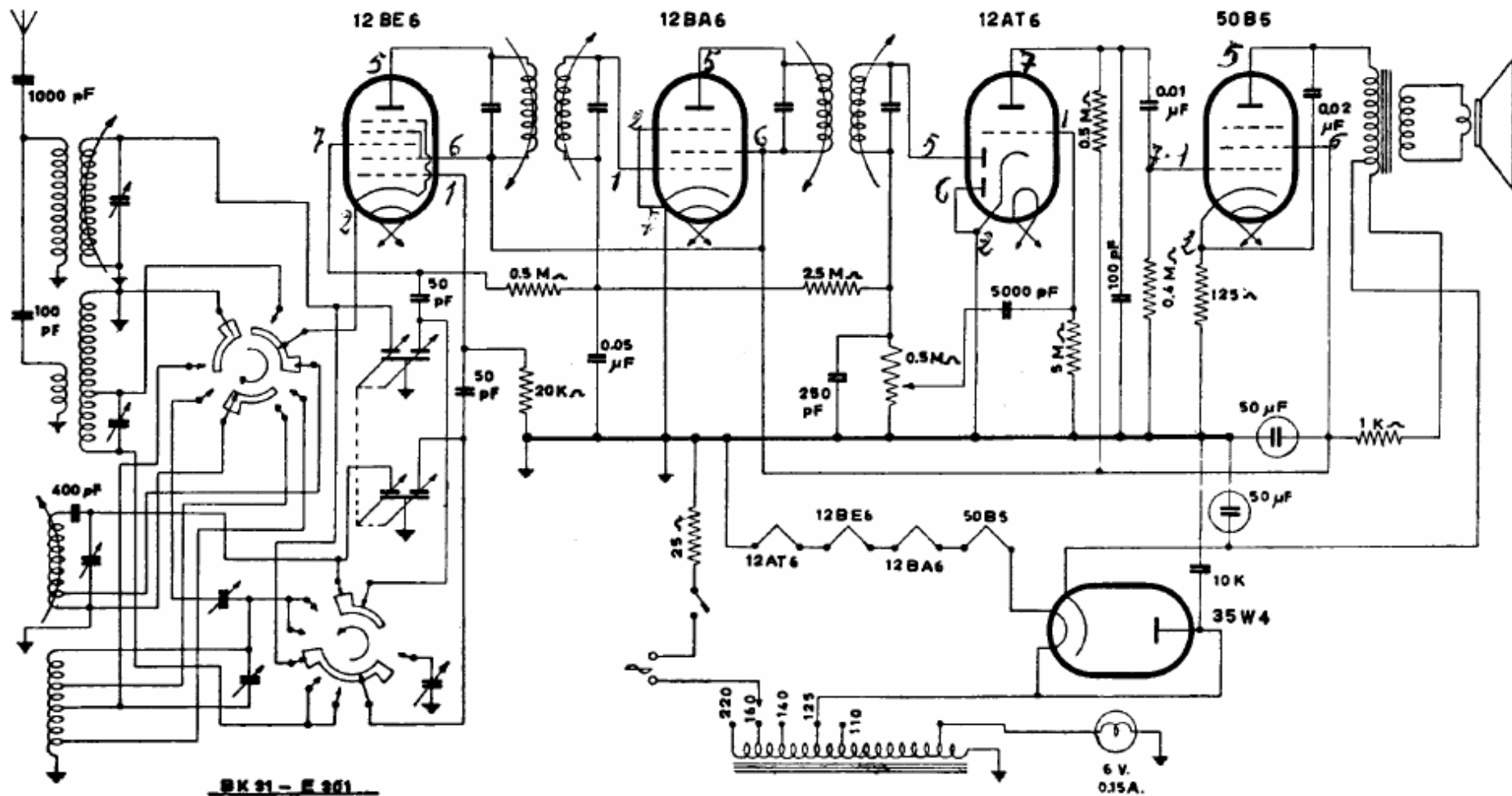
IRRADIO - Modd. BK 31 e E 301. Media frequenza 467 kc. Potenza d'uscita 4 watt.
